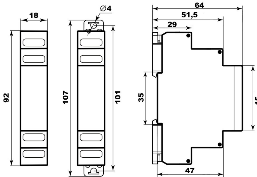
Рис. 3 — Габаритные размеры
